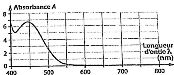
Spectre d'absorption d'une solution de K_2CrO_4
