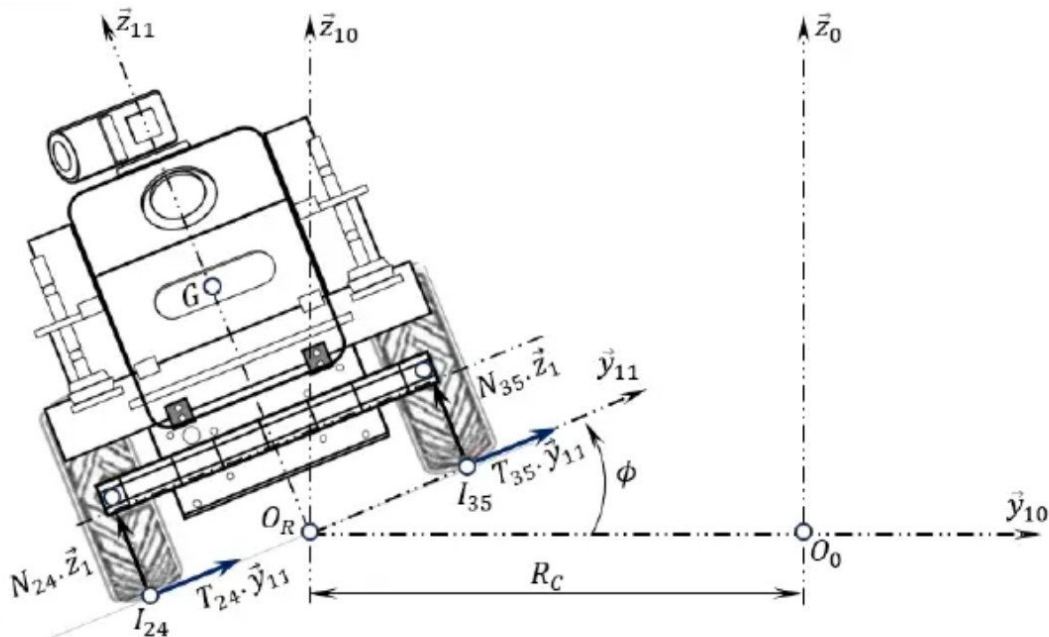
Figure 18 : Configuration du robot dans le plan de l'étude
