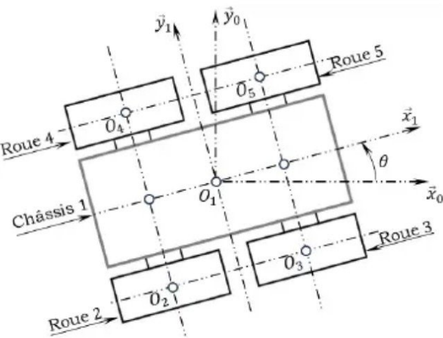
Figure 17 : Repérage et paramétrage du robot.
