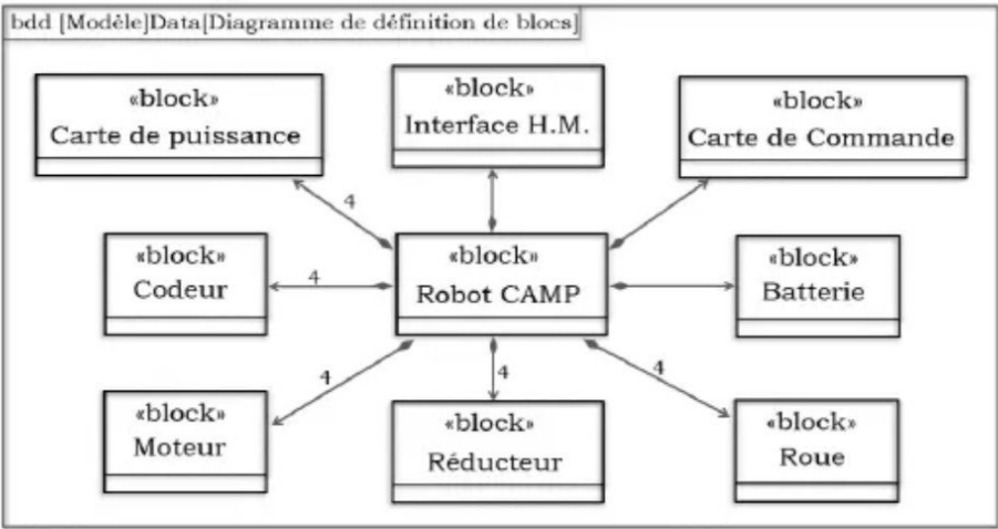
Figure 4 : Diagramme de définition de blocs partiel
