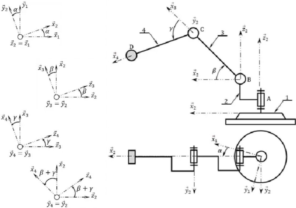
Figure 11 : Schéma cinématique du manipulateur
