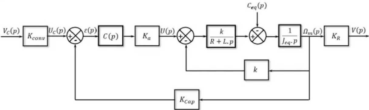
Figure 6 : Schéma-blocs de l'asservissement en vitesse
