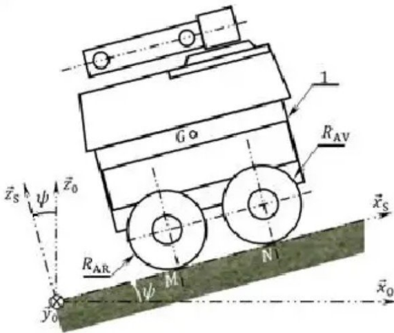
Figure 15 : Robot en mouvement sur un sol incliné
