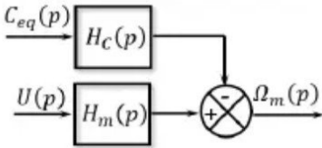
Figure 8 : Schéma équivalent du moteur
