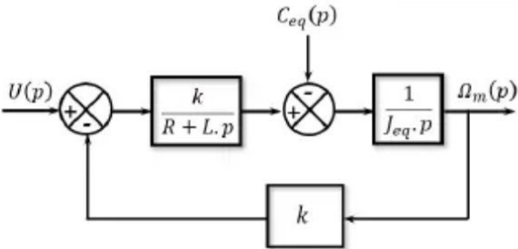
Figure 7 : Schéma blocs du moteur
