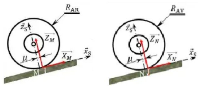
Figure 16 : Modélisation du contact roue/sol
