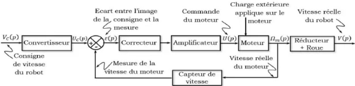
Figure 5 : Schéma fonctionnel de l'asservissement en vitesse d'un des moteurs
