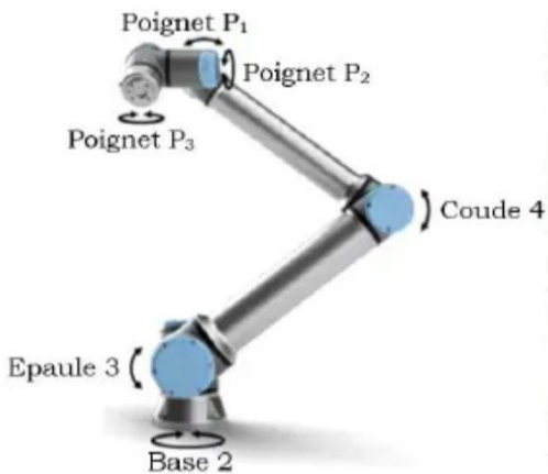
Figure 2 : Manipulateur Ur
