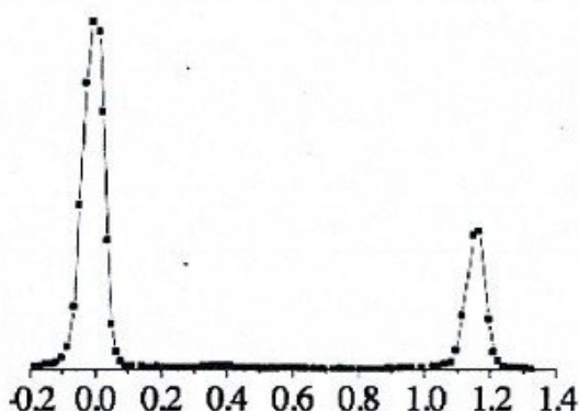
Figure 2-7 : Signal détecté en fonction de l'angle \theta de déflexion.
