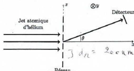
Figure 2-6 : Diffraction d'un jet d'hélium par un réseau.
