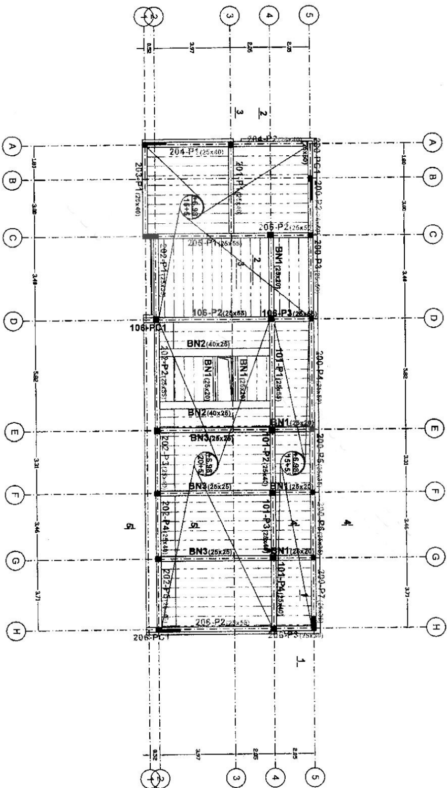
Plancher Terrasse
