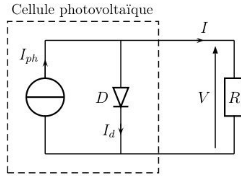
FIGURE 2 – Schéma électrique équivalent d'une cellule photovoltaïque sans pertes.
