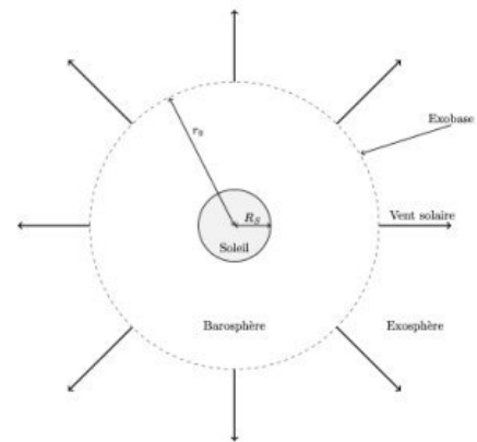
Figure 2 : Schéma modélisant le Soleil et la couronne solaire ( r_0 \approx 5R_s ).
