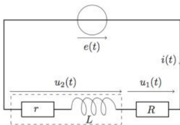
Figure 2.2 : circuit de mesure de L
