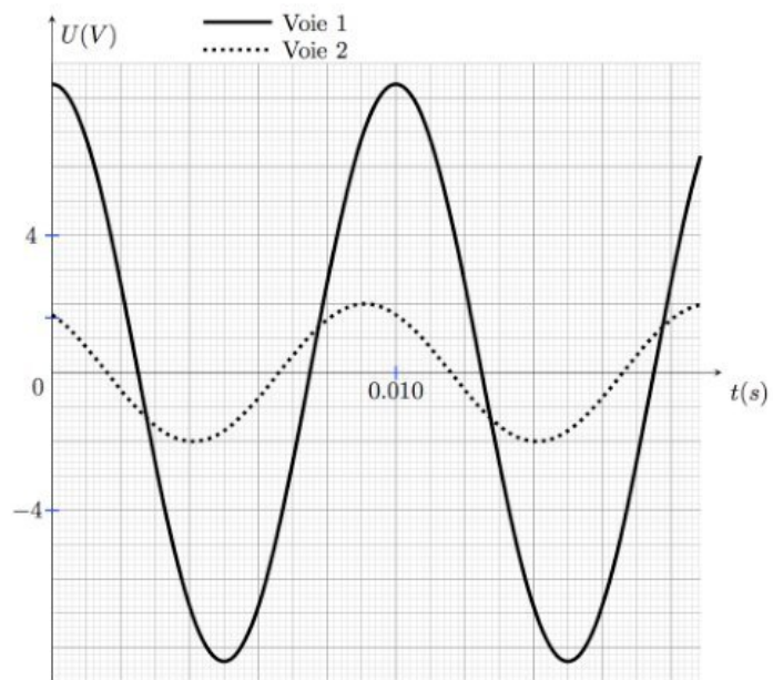
Figure 2.3 : chronogrammes
