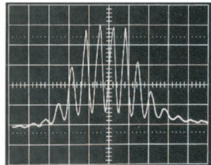
Figure 4 : Tension en sortie du photodétecteur ( 1 \text{ V/div} et 1 \mu\text{s/div} ).
