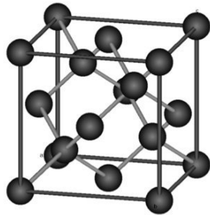
Figure : maille élémentaire de germanium
