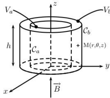
Figure 2: Milieu conducteur entre deux cylindres.
