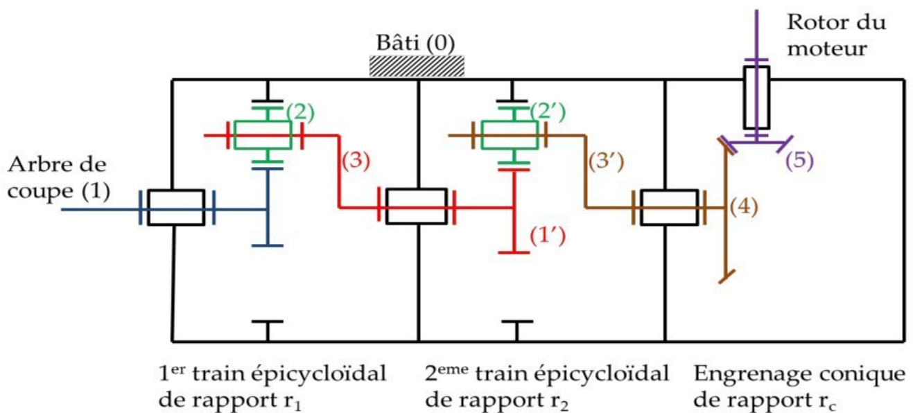
Figure 6 : Réducteur
