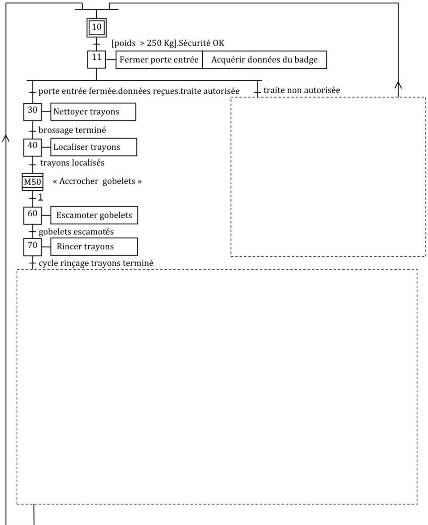
Figure R2 : Grafcet G_1 de gestion des tâches à compléter
