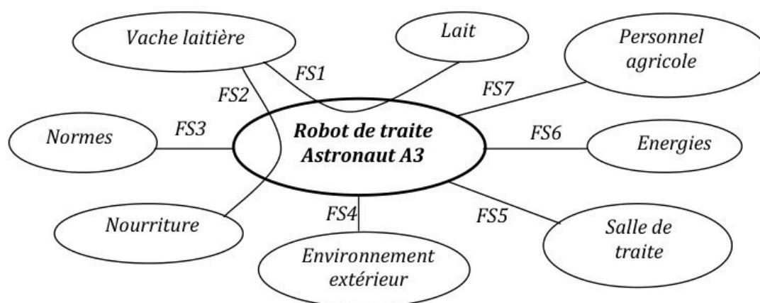
Figure 3 : Diagramme partiel des inter-acteurs du robot de traite Astronaut A3.
