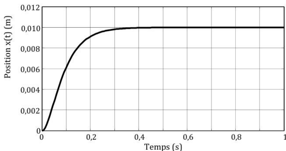
Figure 17 : La position du chariot 1 pour un échelon de position de 0,01 \text{ m} avec les trois boucles.
