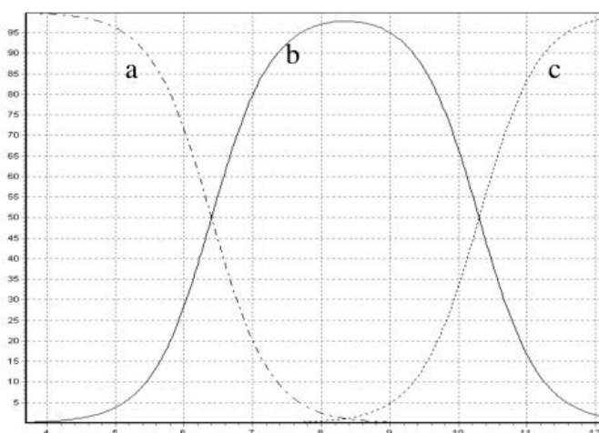
Figure 1 : Diagramme de distribution des espèces acido-basiques dérivées de \text{CO}_{2(\text{aq})}
