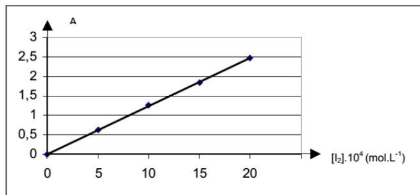
Figure 3 : L'absorbance en fonction de la concentration des solutions en I_2
