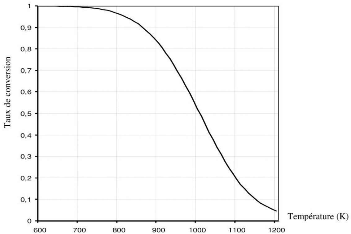
Figure 1 : Taux de conversion \alpha en fonction de la température
