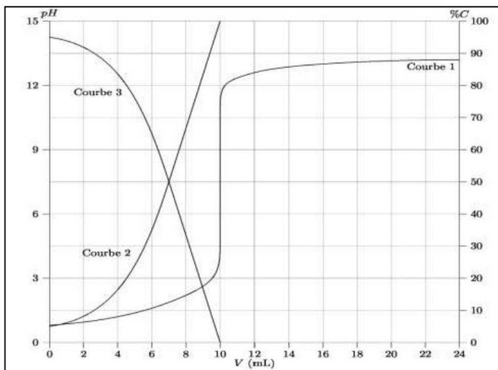
Figure 2 : Titrage de l'acide sulfurique
