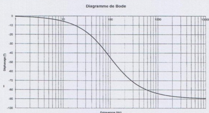
Figure 7: Diagramme de Bode en phase
