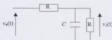
Figure 8: Filtre
