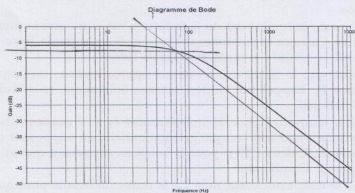
Figure 6: Diagramme de Bode en gain
