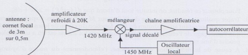
Figure 5: Simulation d'un élément de radiotélescope
