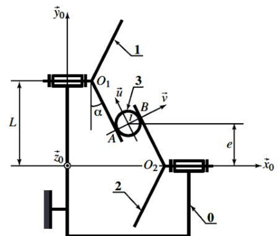
Figure 2 : variateur de vitesse à bille
