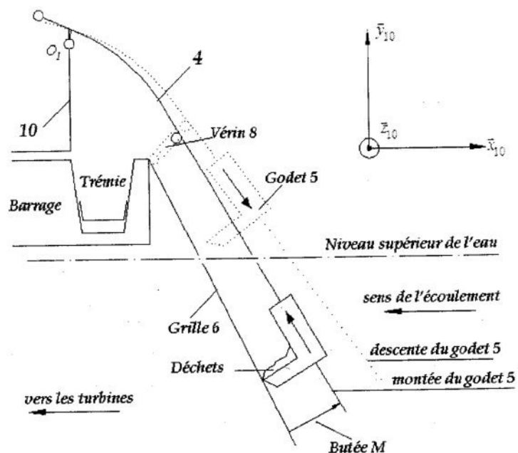
Figure 1-b : Schéma d'implantation
