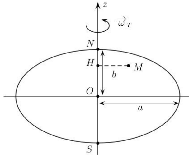
FIGURE 4 – Terre ellipsoïdale.
