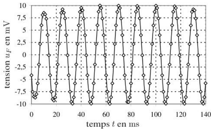
Figure 4: Exemple d'enregistrement de la tension DOPPLER.
