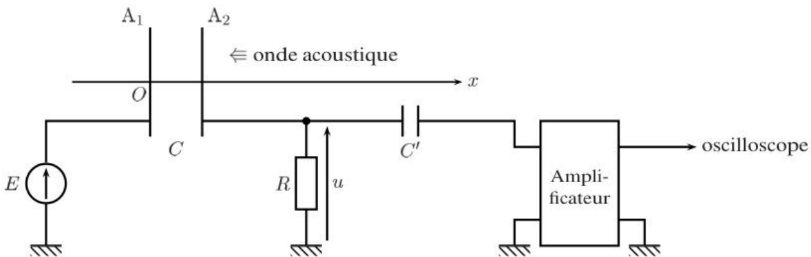
Figure 1: Montage d'un microphone électrostatique.
