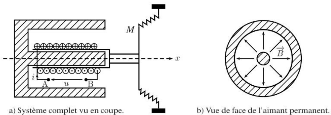
Figure 2: Haut-parleur électrodynamique.
