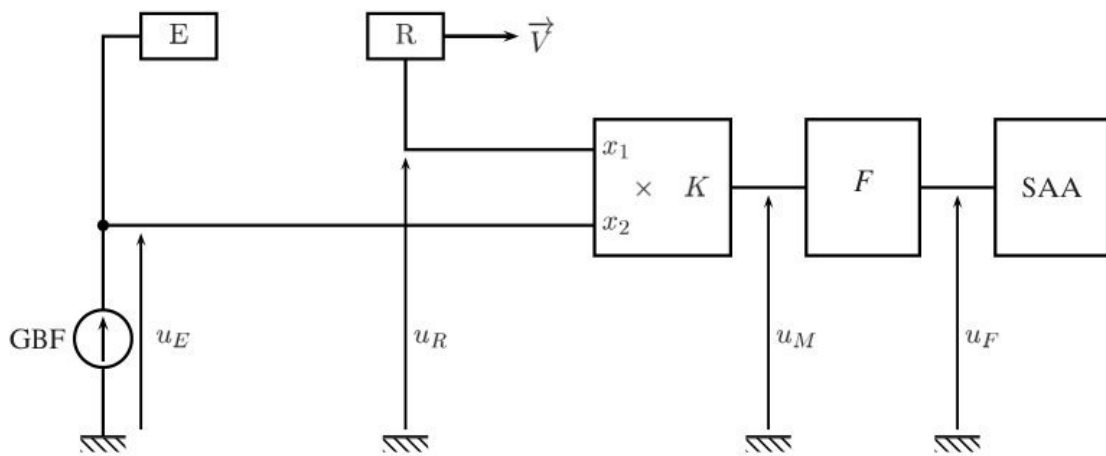
Figure 3: Dispositif de mesure d'une vitesse de translation par effet DOPPLER.
