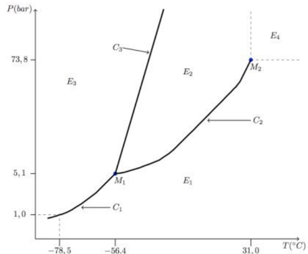
Figure 1 : Diagramme d'état du CO_2
