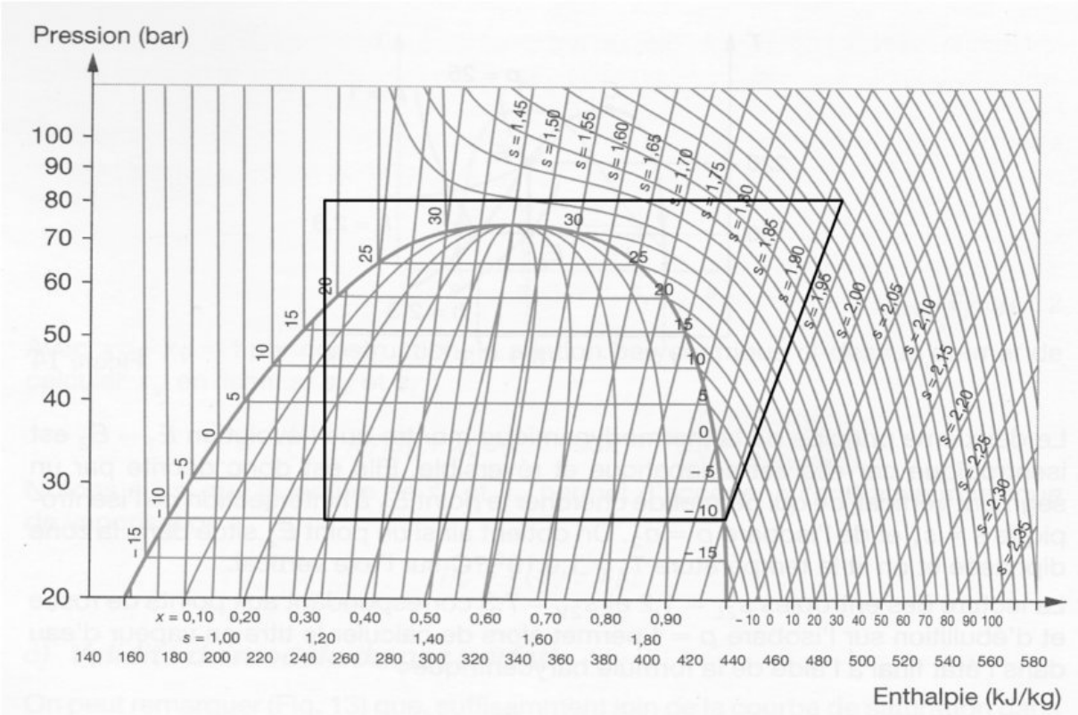
Figure 3 : Diagramme (P,h) des frigorigènes du \text{CO}_2
