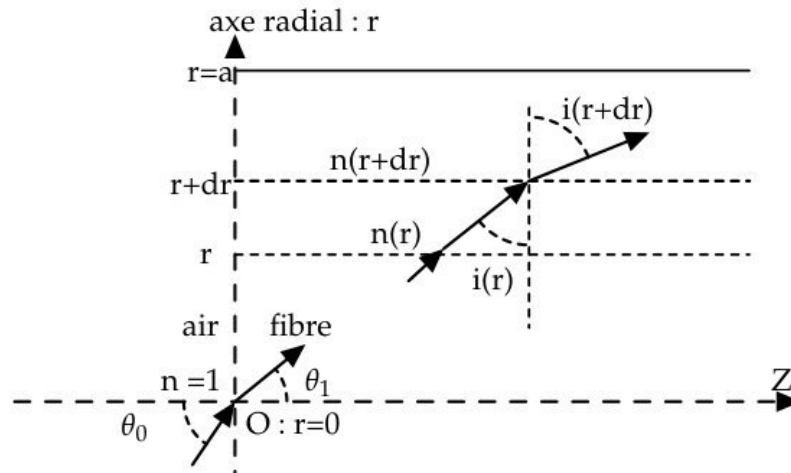
Figure 6 – Fibre à gradient d'indice
