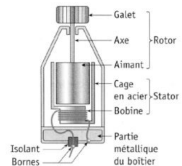
Figure 5 : Dynamo de vélo
