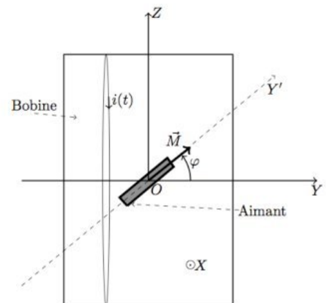
Figure 6 : Schéma de principe d'un alternateur de vélo
