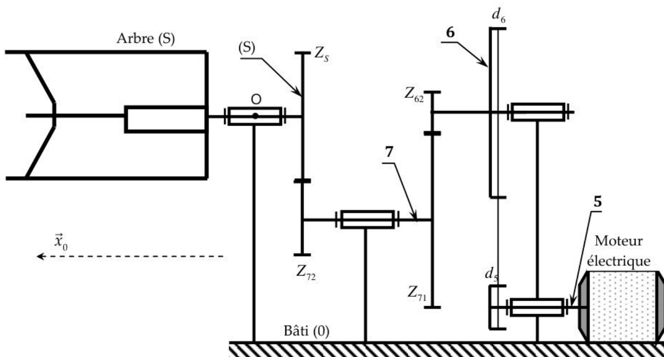
Figure 10 : Schéma de la transmission de puissance de rotation de l'arbre.
