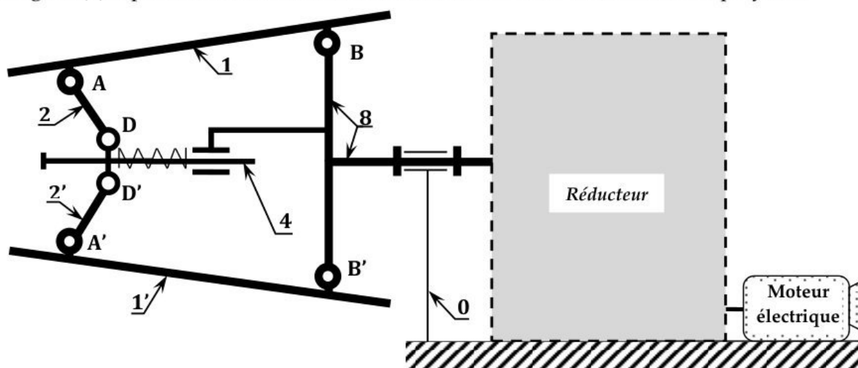
Figure 5 : Schéma du système d'extraction de polyane.
