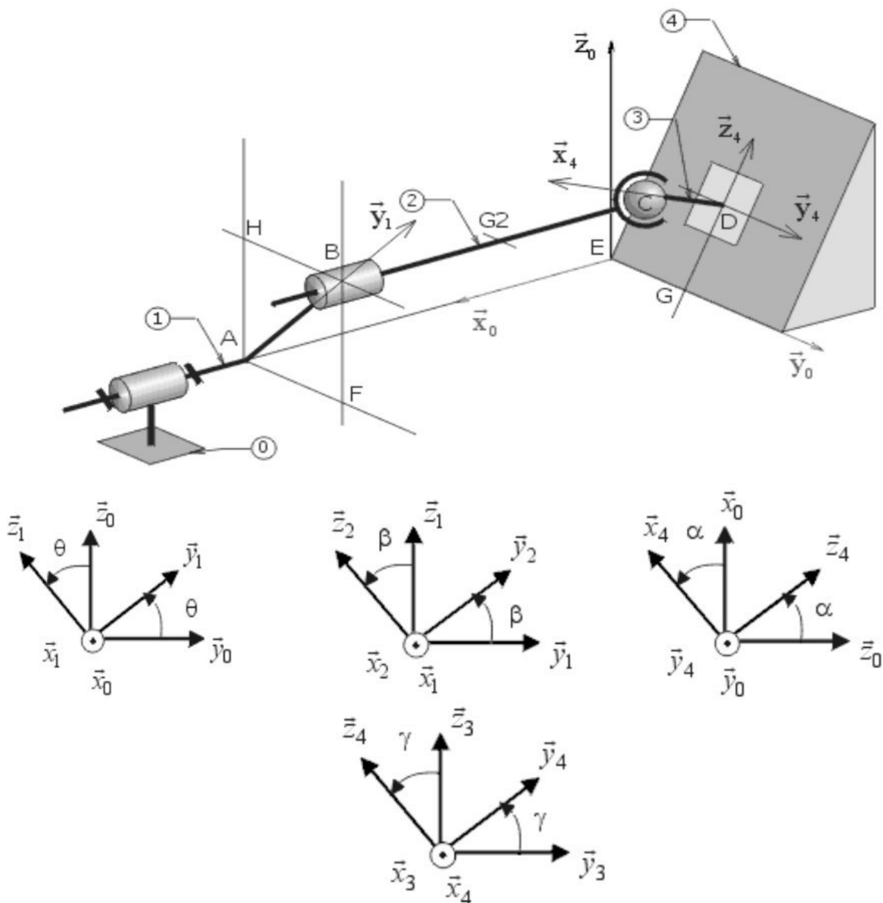
Figure 3 : Schéma cinématique de la pompe
