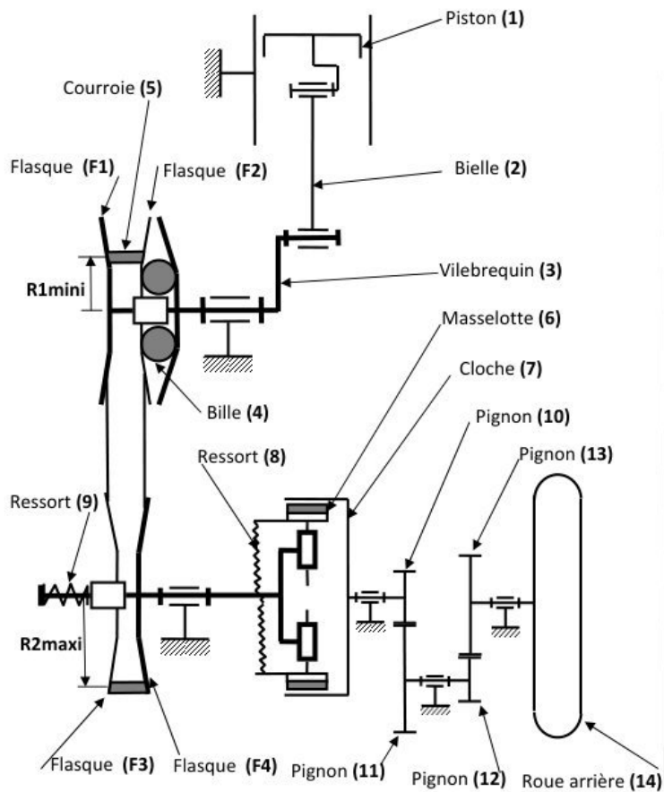
Figure 1 : Phase de ralenti
