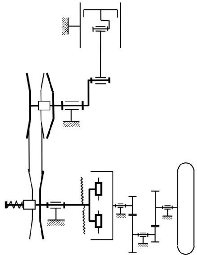
Figure 2 : Phase de glissement dans l'embrayage
