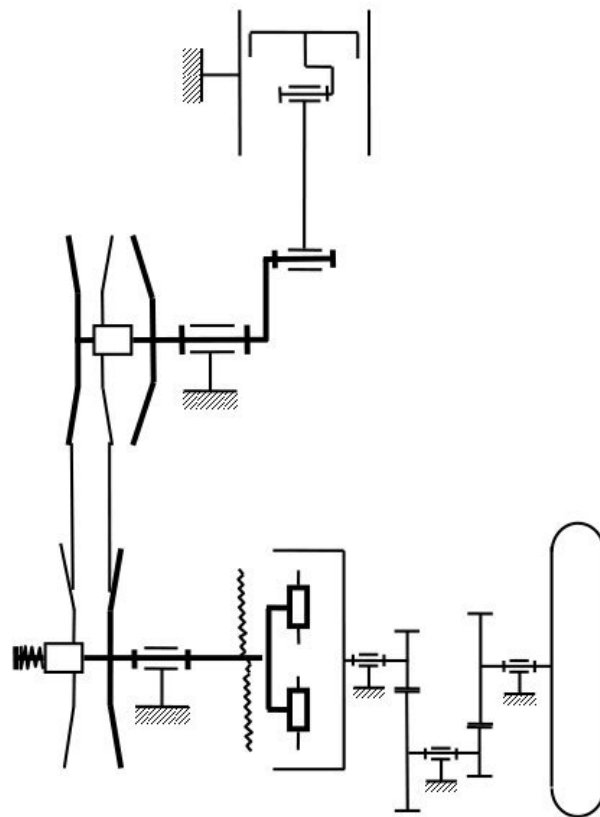
Figure 4 : Phase de vitesse maximale du scooter
