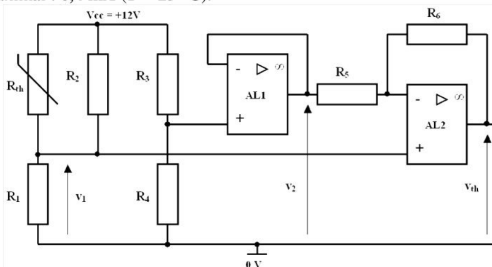
Figure 6 - Capteur de température.
