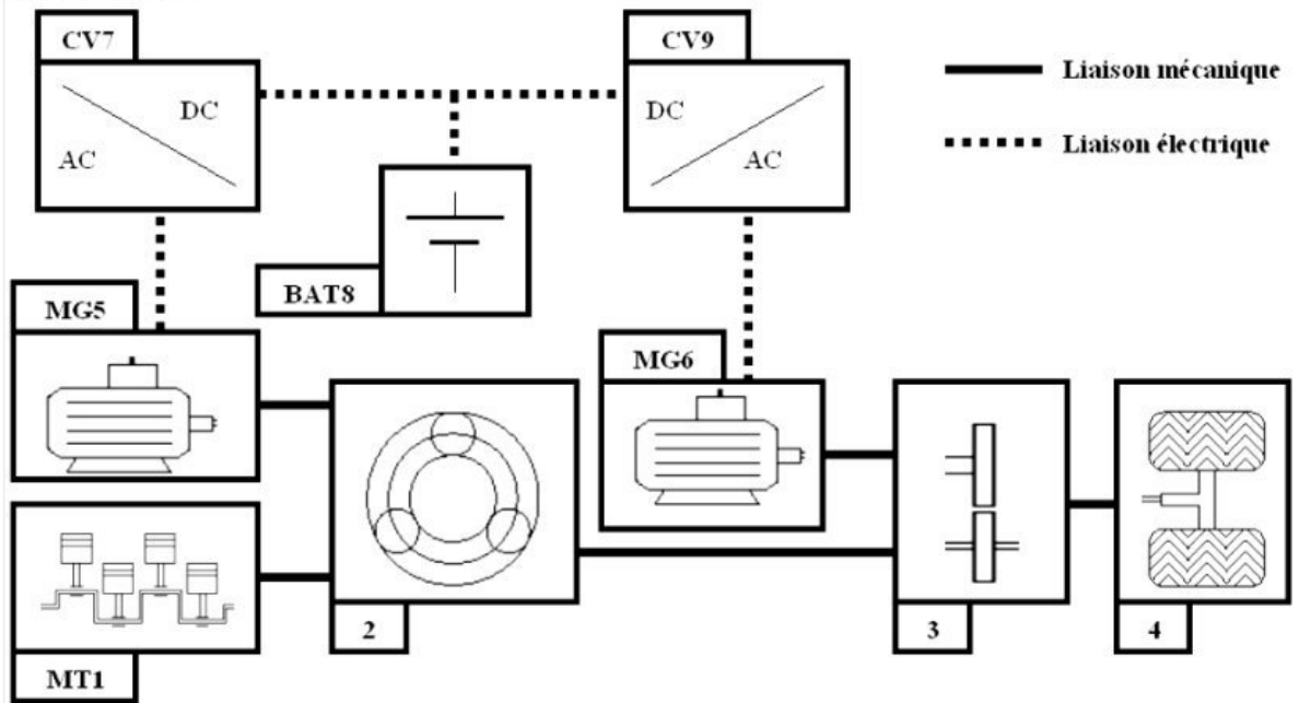
Figure 1 - Chaîne simplifiée de transmission des énergies.
