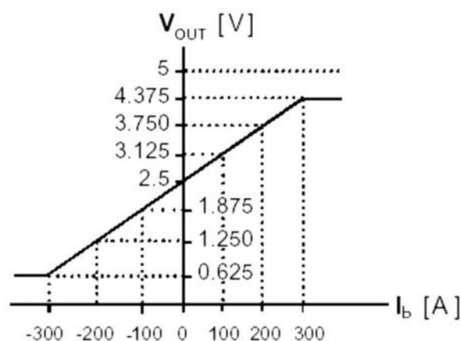
Figure 7 :Caractéristique de sortie du capteur
