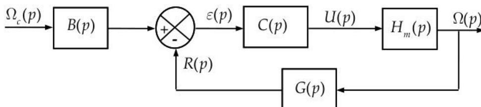
Figure 14 : Schéma- bloc de l'asservissement en vitesse.
