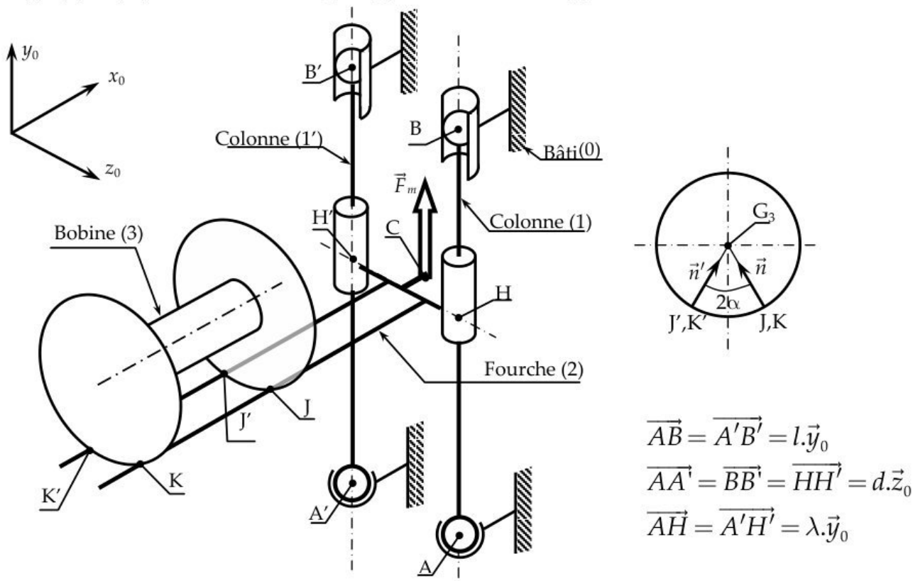
Figure 2 : Schéma cinématique du mécanisme élévateur+bobine
