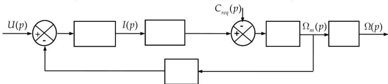
Figure 13 : Schéma- bloc de l'ensemble moteur + charge.
