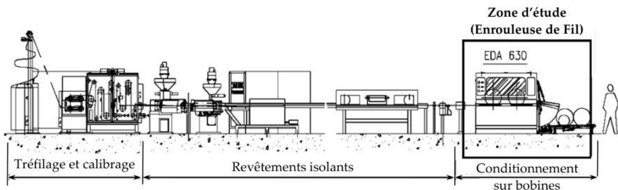
Figure 1 : ligne de production du fil
