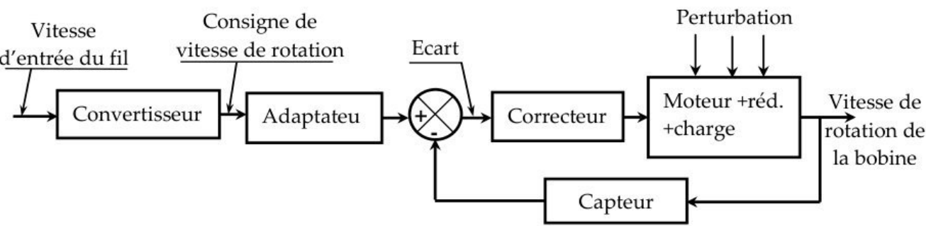
Figure 12 : Structure de l'asservissement.
