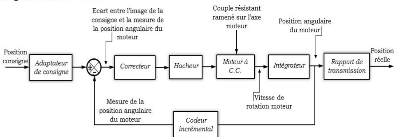
Figure 5 : schéma bloc fonctionnel de l'asservissement
