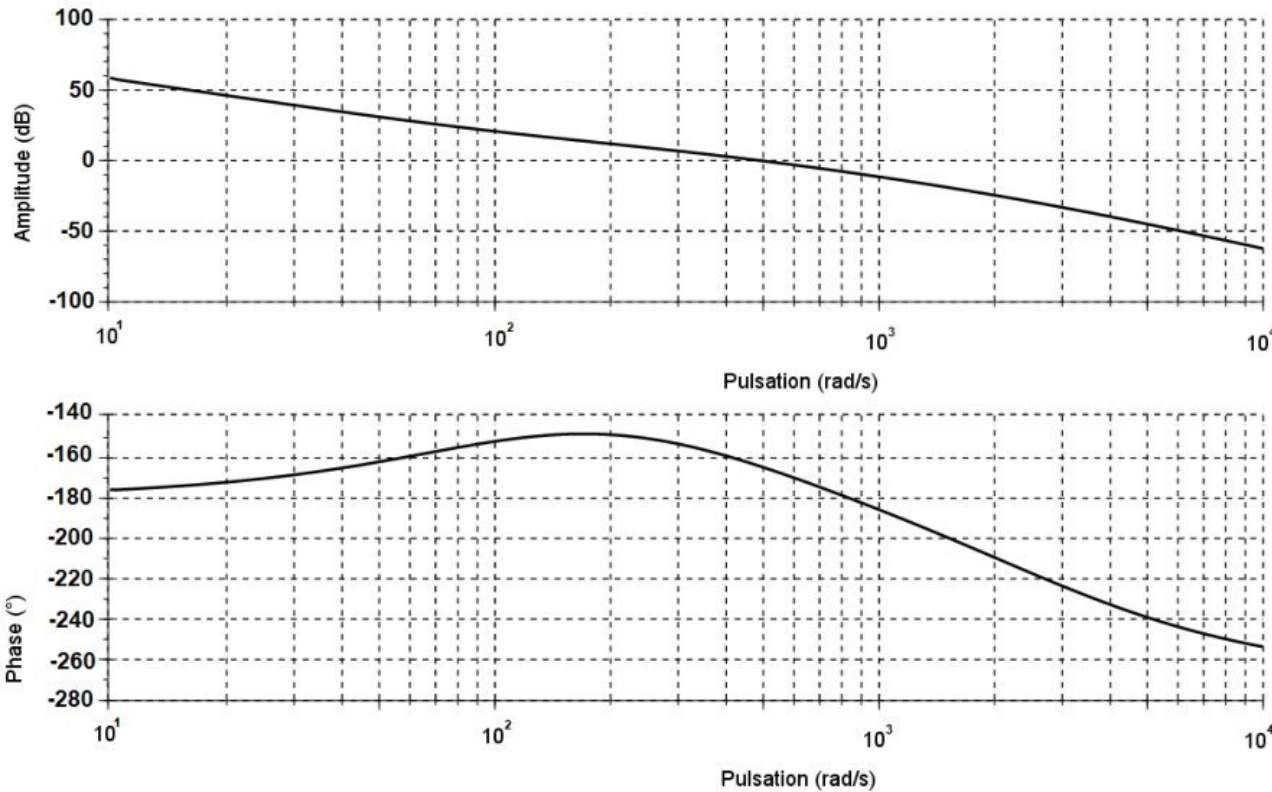
Figure R4 : Diagramme de Bode de la FTBO corrigée pour K_i = 1 .
