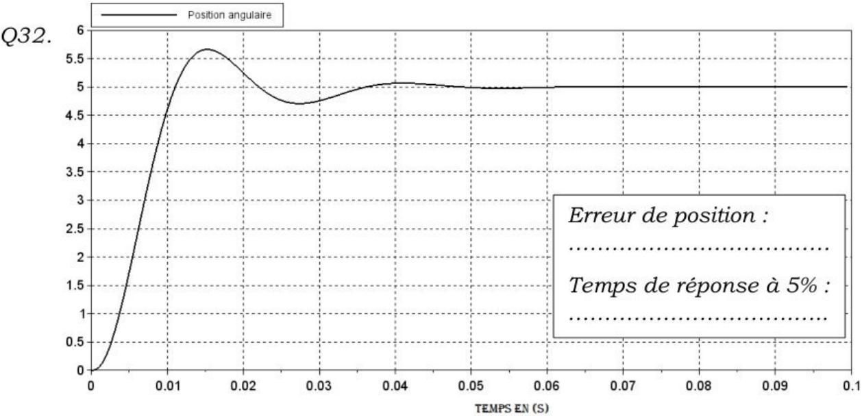
Figure R5 : réponse indicielle à un échelon de position de 5^\circ
