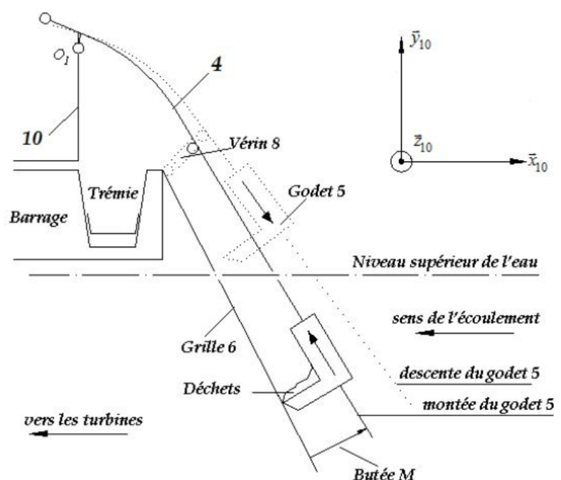
Figure 1-b : Schéma d'implantation
