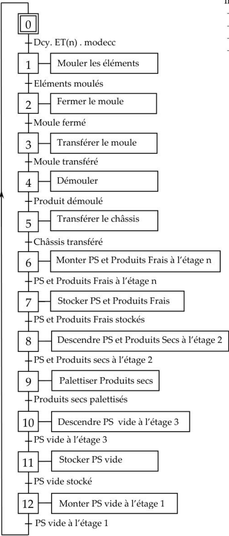
Grafcet de coordination des tâches en production normale, en mode « cycle à cycle»
