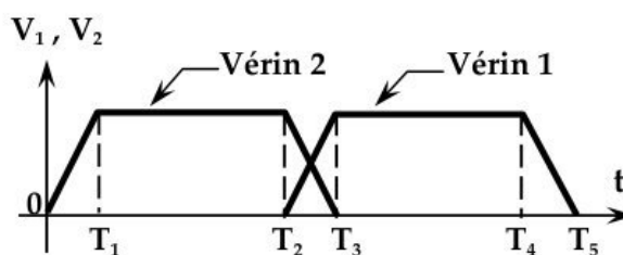
Figure 1 : Lois des vitesses des vérins 1 et 2
