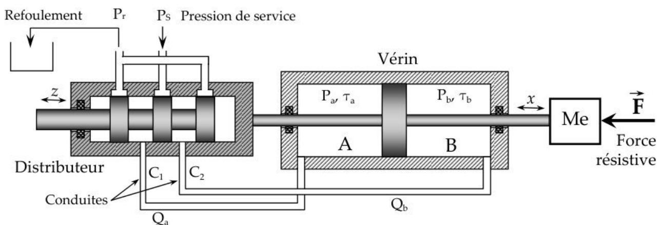
Figure 3 : Vérin hydraulique à commande directe.
