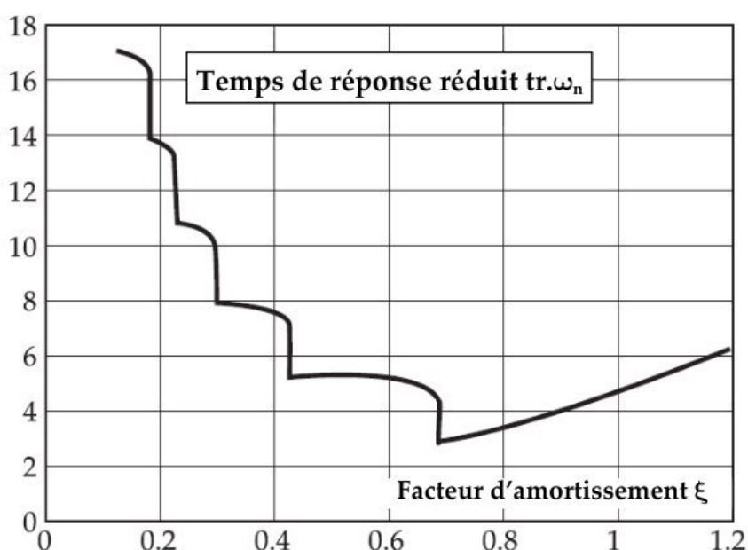
Figure 5 : Abaque du temps de réponse réduit du 2 nd ordre : tr.\omega_n = f(\xi)
