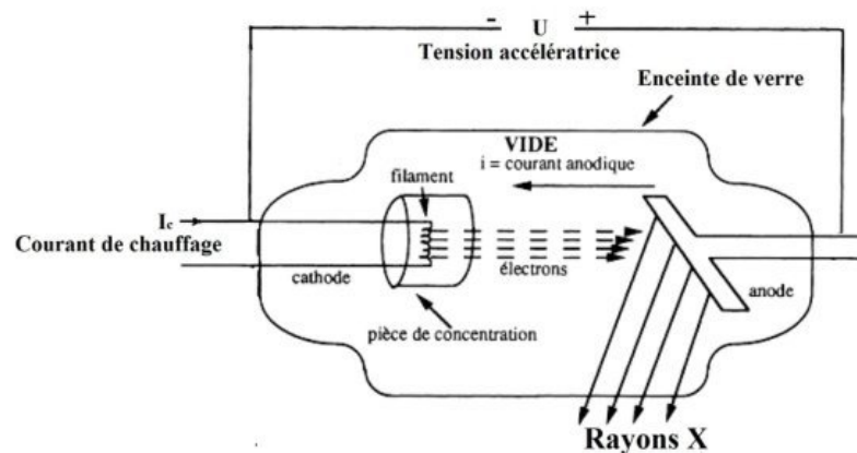
Figure 1 – Principe de production des rayons X : tube de Coolidge
