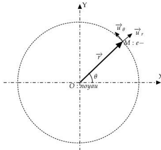
Figure 3 – L'atome d'hydrogène
