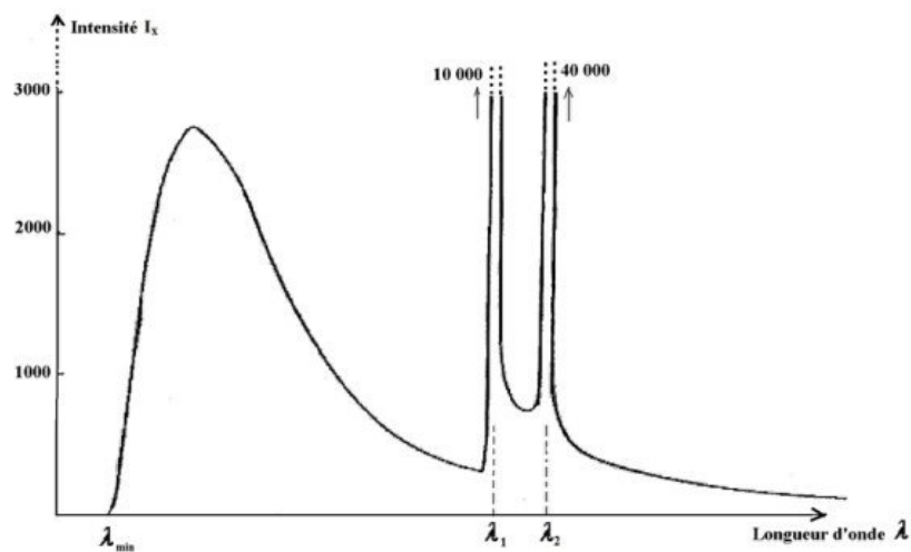
Figure 2 – Spectre de rayonnements émis par une anode en cuivre sous une tension de 40 kV
