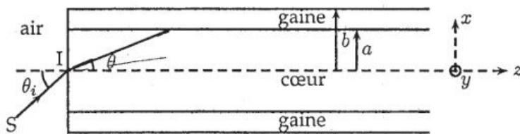
Fig 2 : Modèle simplifié d'une fibre optique à saut d'indice.
