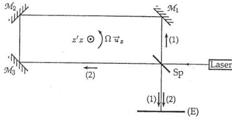
Fig 5 : Interféromètre de SAGNAC.
