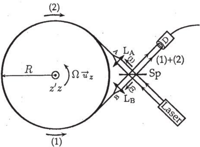
Fig 6 : Schéma de principe d'un gyromètre à fibre optique.
