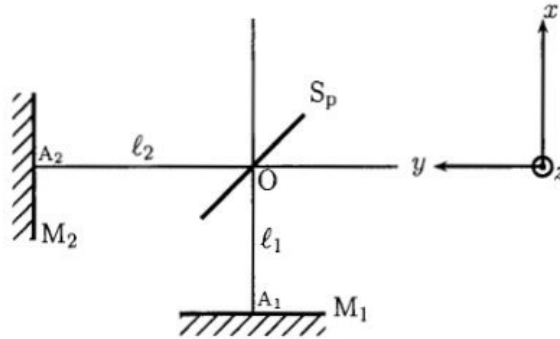
Figure 1: Modèle d'interféromètre de MICHELSON.
