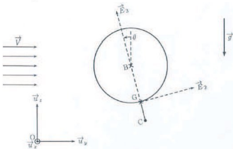
Fig 2 : Ballon-sonde en mouvement dans le champ de pesanteur.
