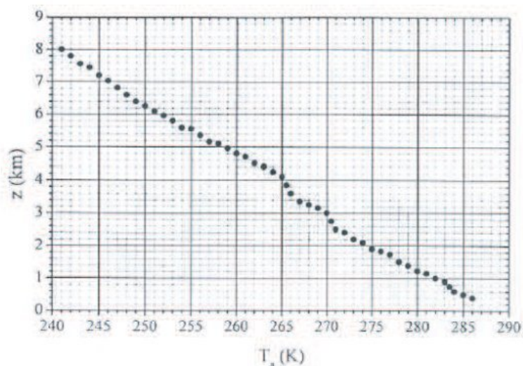
Fig 1 : Profil vertical de température mesuré par le ballon-sonde.
