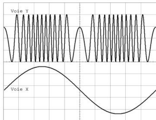
(b) Oscillogramme obtenu pour f = f_2 .
