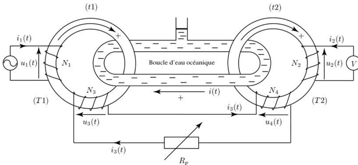
Figure 1: Dispositif de mesure de la conductivité de l'eau océanique par induction.
