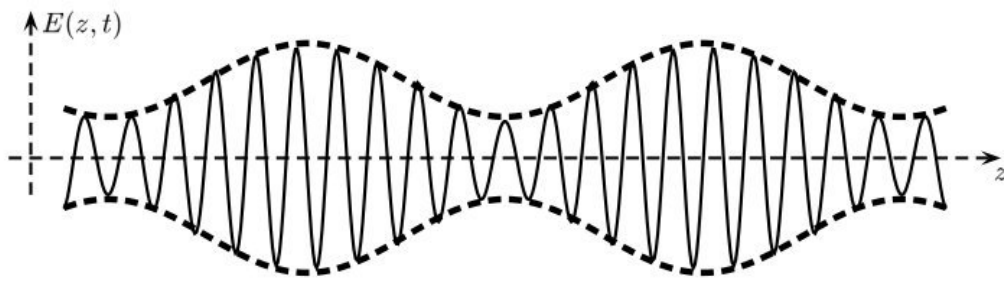
Figure 6 : Représentation schématique des variations du champ électrique dans le guide.
