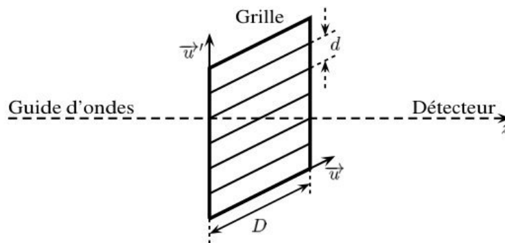
Figure 4 : Grille métallique.
