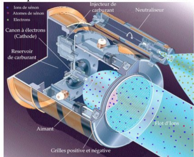
Figure 2 : Schéma du moteur ionique
