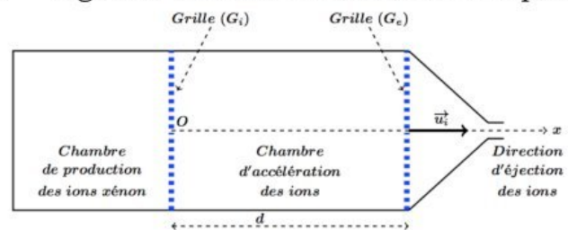
Figure 3 : Principe du moteur ionique
