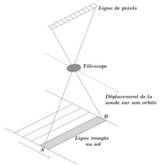
Figure 5 : Principe de l'imagerie par sonde « Push-broom »
