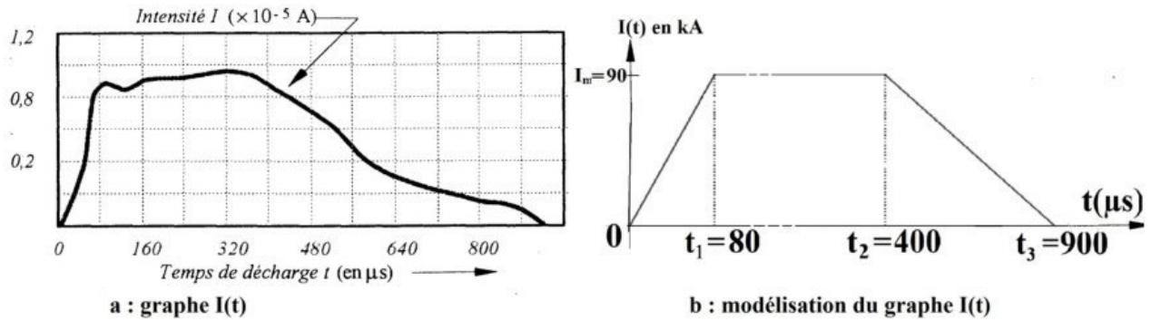
Figure 6 – Intensité du courant lors d'un éclair
