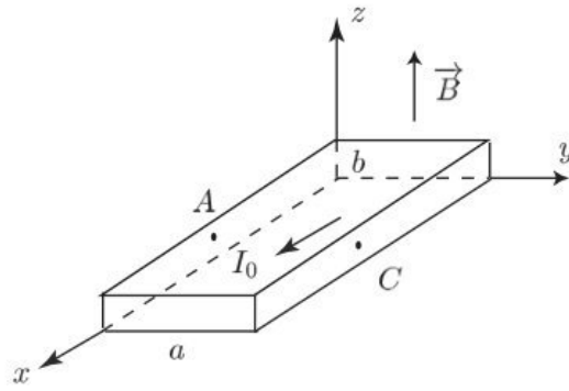
FIG. 1 – Ruban conducteur dans un champ magnétostatique
