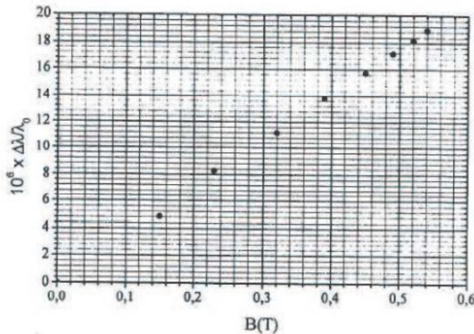
Fig 1 : Variation de la longueur d'onde avec le champ magnétique.
