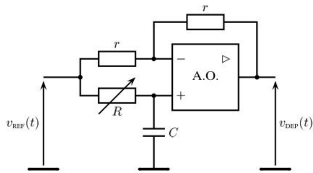
Figure 5: Circuit déphaseur à amplificateur opérationnel.
