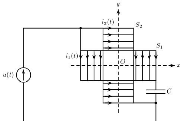
Figure 3: Deux solénoïdes croisés insérés dans un circuit électrique. Pour des raisons de clarté, les spires ne sont pas représentées dans la partie commune centrale.
