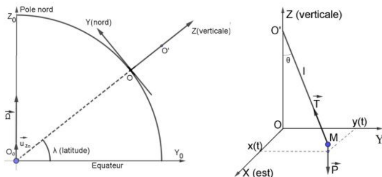
Figure 2 – Pendule de Foucault dans le référentiel Terrestre
