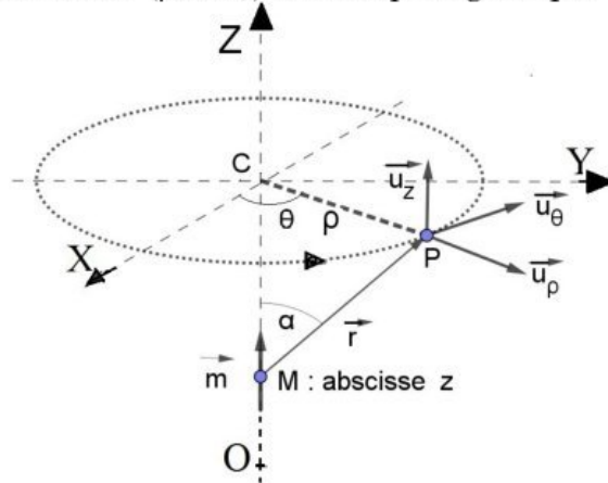
Figure 5 – Champ magnétique crée par un dipôle magnétique
