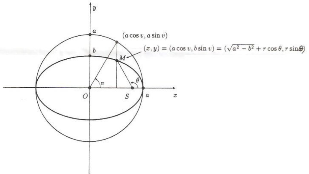
Figure : Ellipse de Kepler et anomalie excentrique v .
