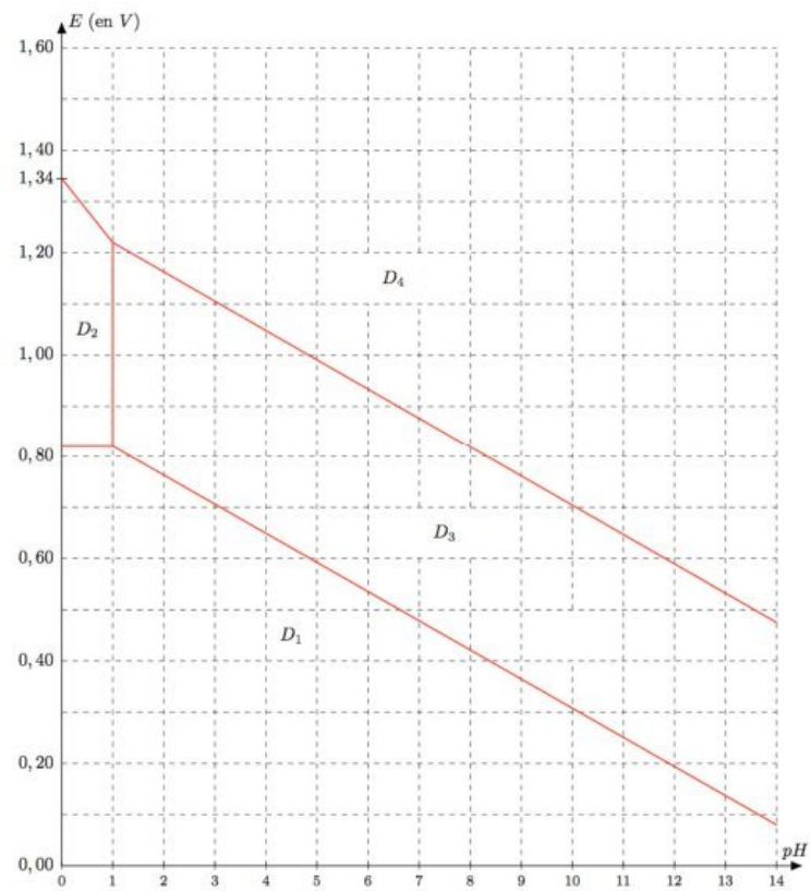
Diagramme potentiel-pH du palladium à 25^\circ C
