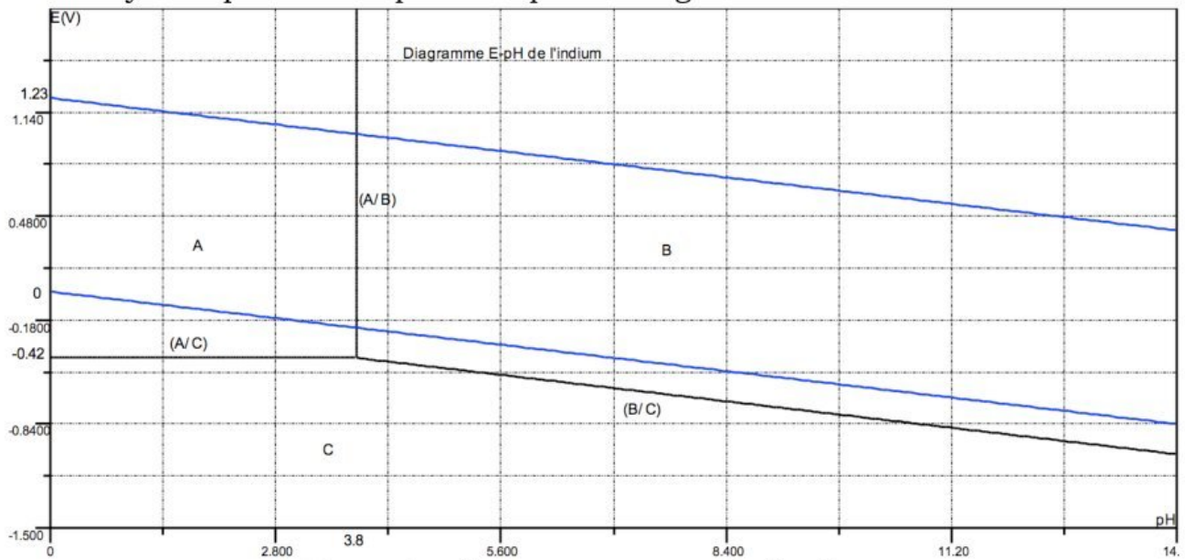
Figure 2 : diagramme E - pH de l'indium
