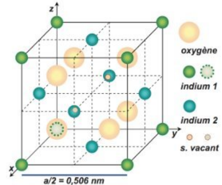
Figure 1-2 : un huitième de la maille In_2O_3
