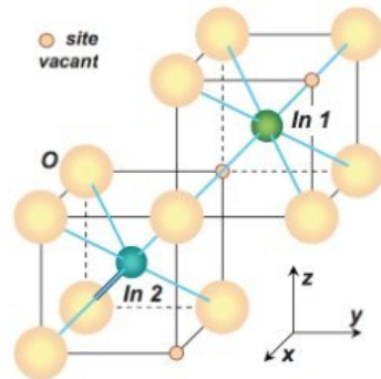
Figure 1-1 : motif élémentaire In_2O_3 , sites vacants et 2 types d'ion indium
