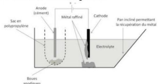
Figure 3 : Électroraffinage de l'indium
